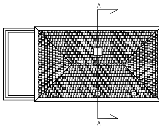
Pianta copertura stato di progetto
