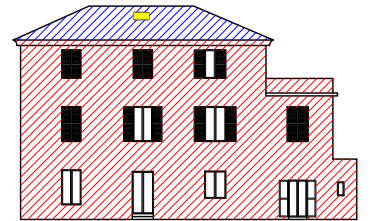
Prospetto sud sovrapposizione
