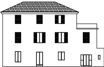
Prospetto sud stato attuale
